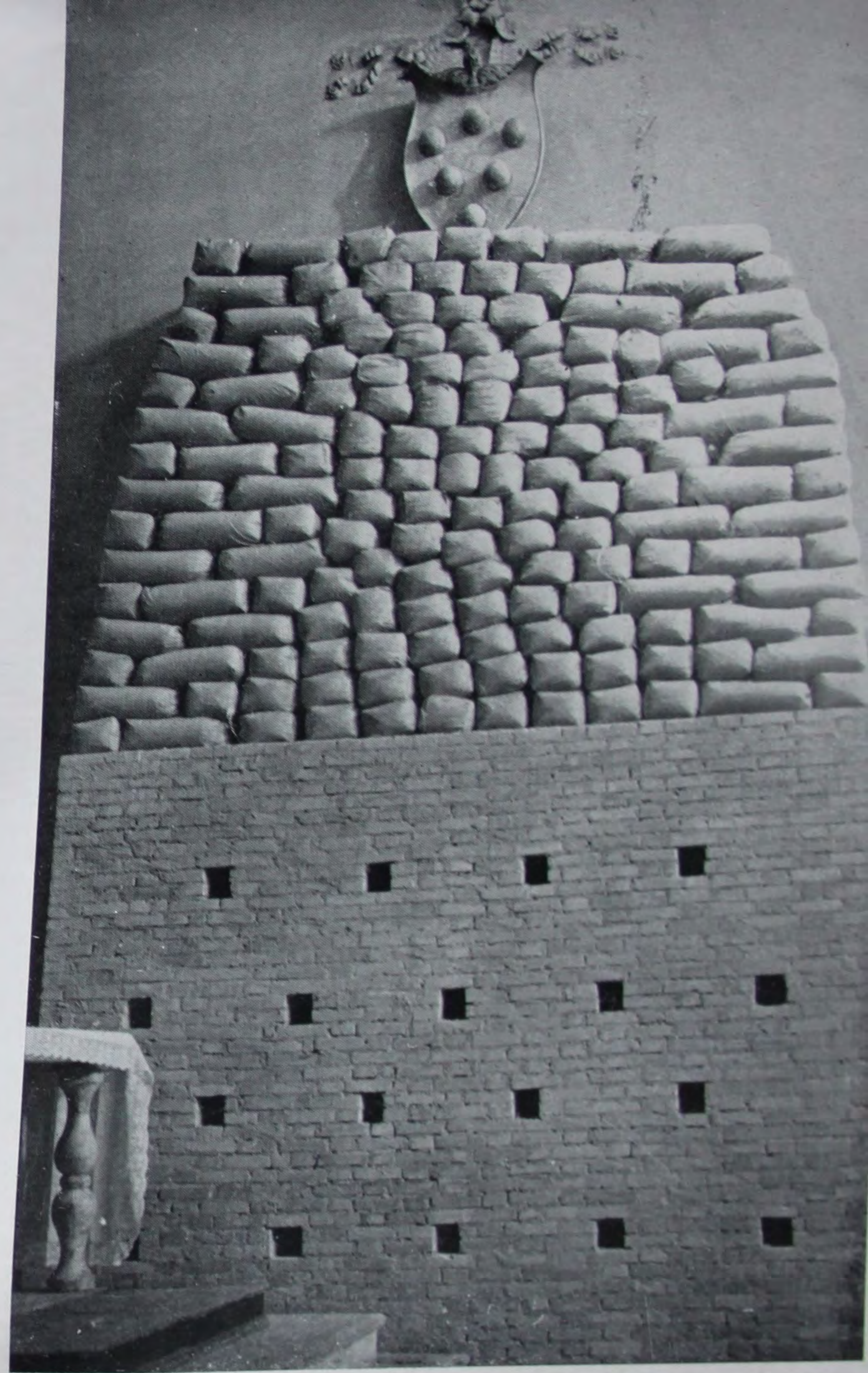
FIRENZE - Chiesa di San Lorenzo. Armature per la protezione della Cantoria di Donatello e della tomba medicea del Verrocchio.
