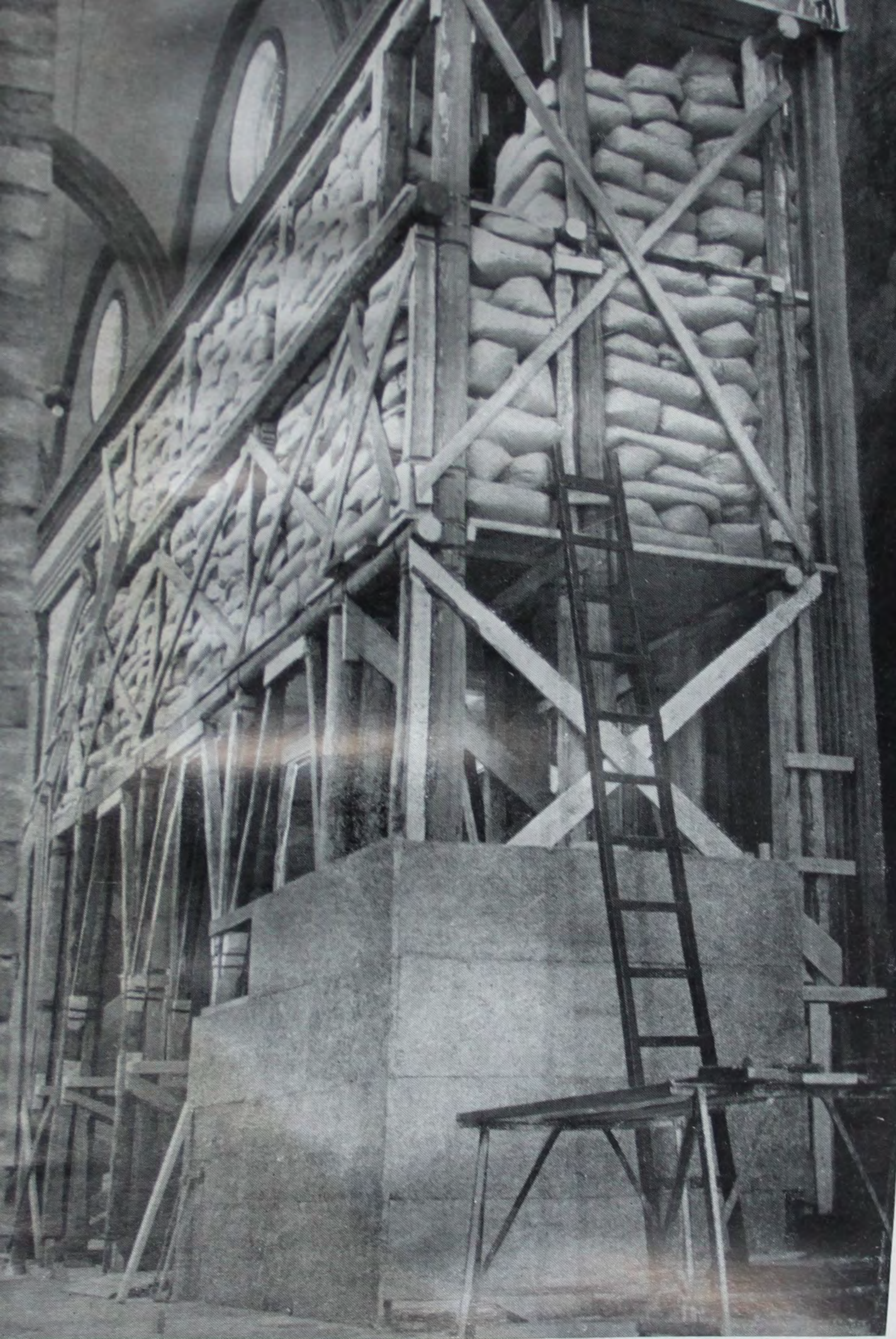
FIRENZE - Chiesa di San Lorenzo. Armature per la protezione della Cantoria di Donatello e della tomba medicea del Verrocchio.
